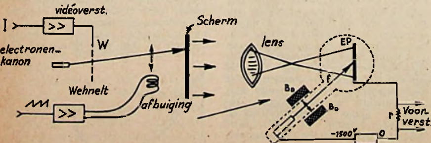
Principeschema van de definitie-transformator bij de Télévision-Française. Links: de ontvanger met de ene definitie; rechts: de iconoscoop met de andere definitie. Als medium het nalichtende ontvangerscherm.
