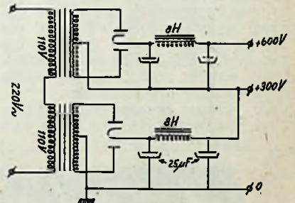
Fig. 6. Serieschakeling van twee identieke dubbelphasige gelijkrichters wordt tegenwoordig in de eenvoudige oscillografen toegepast.
