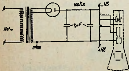
Fig. 1. Eenvoudige wijze voor de opwekking van de versnellingsspanning voor een kathodestraalbuis, met enkelvoudige trafo.
