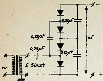
Fig. 8. Cascadevermenigvuldiger. De spanning wordt met het aantal cellen trapsgewijze verhoogd.
