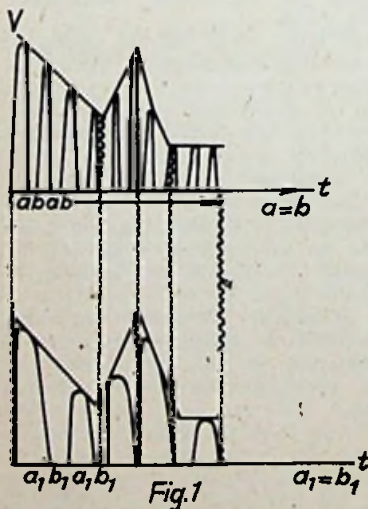
Zelfde videosigitaal op verschillende golflengte. De definitiefrequentie moet slechts enige malen lager liggen dan de draaggolf. (In deze zin voldoet de figuur dus niet!)
