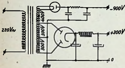
Fig. 4. Veel gebruikelijke schakeling in de oudere oscillografen. Een extra spanningswikkeling op de voedingsrafo staat in serie met een helft van de andere secundaire wikkeling.
