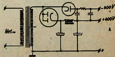
Fig. 3. Spanningsverdubbelschakeling.
