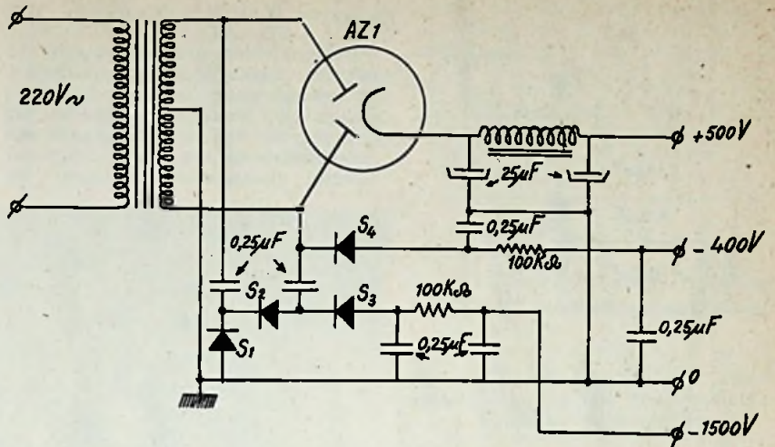
Fig. 7. Een andere wijze van spanningsvermenigvuldiging, die vaak toegepast in door radio-amateurs gebouwde TV-ontvangers.
