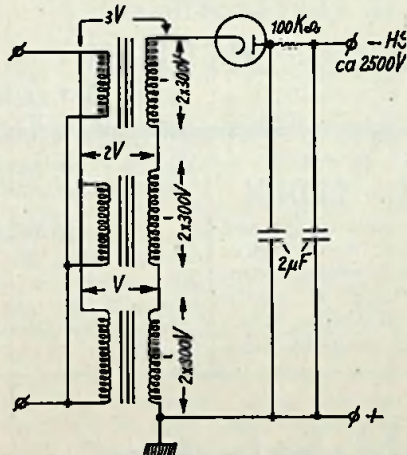
Fig. 2. Serieschakeling van trafo's voor het verkrijgen van een hoge spanning kan moeilijkheden geven met de isolatie. De spanning tussen gestel en wikkelingen neemt met de serieschakeling toe.
