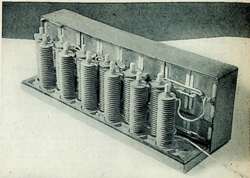
Fig. 9. Experimentele uitvoering van een cascadevermenigvuldiger. Bij een ingangswisselspanning van 220 eff. werd een uitgangsgelijkspanning van iets meer dan 3000 Volt verkregen bij een belasting van 5 mA.
