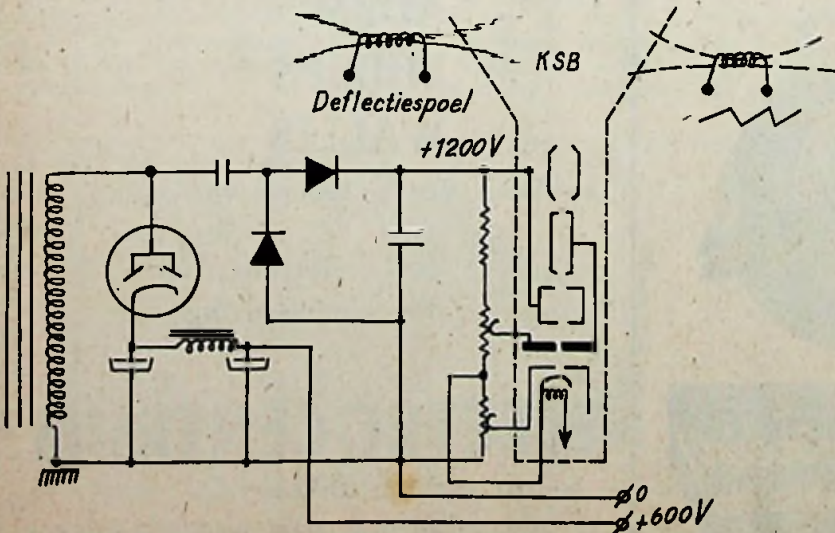
Fig. 5. Een spanningsverdubbelingsschakeling in gebruik bij een electro-magnetische kathodestraalbuis.
